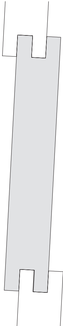
Stülpchalung, beidseitig genutet 20 bis 30 mm
