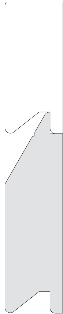
Rhomoid, Nut + Kamm 60° 20 bis 35 mm
