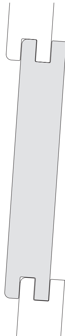
Stülpchalung, beidseitig genutet, gerundet 20 bis 30 mm
