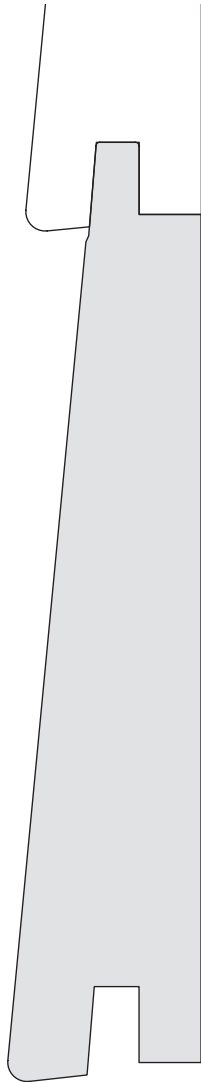
Konische Stülpschalung, Nut + Kamm 15/25 bis 19/34 mm
