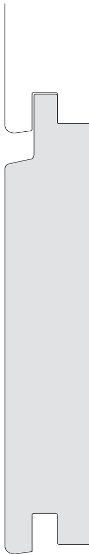
Falzbrett, Nut + Kamm, horizontal 18 bis 25 mm
