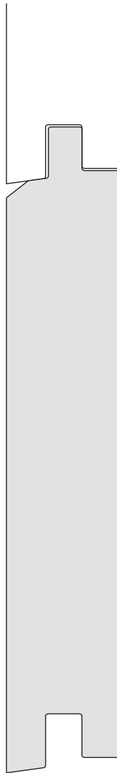
Chaletschalung, Fas 20 bis 35 mm
